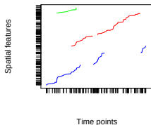
STT: trajectory
